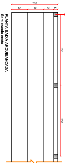
DETALHES ARQUIBANCADA
